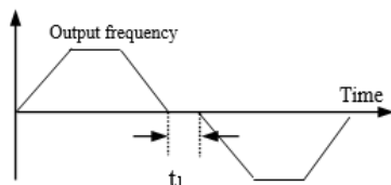
Fig.6-1 Tempo morto FWD/REV
