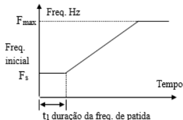
Fig.6-10 Freq. de partida e tempo de duração
