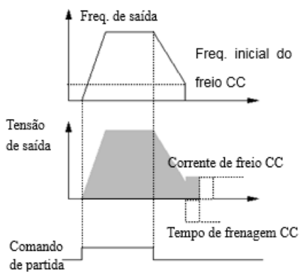
Fig.6-12 Freio de parada CC
