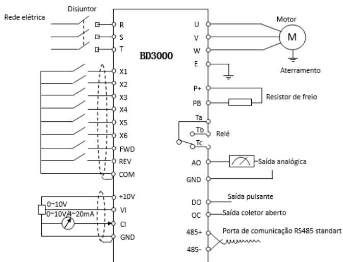
Figura 3-4 Diagrama completo de ligação
