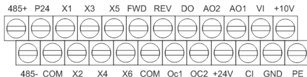
Fig.3-10 Ordem dos terminais CN3 (Inversores acima de 7,5kW)
