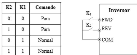
Fig.6-22 Comando 2 fios modo 2
