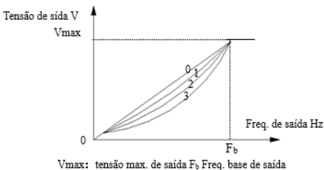
Fig. 6—7 Curvas V/F
