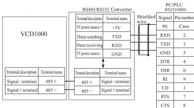
Fig. 3-11 Conexão da porta RS485/RS232
