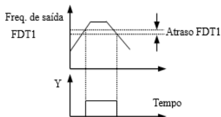
Fig. 6-27 Detecção do Nível de frequência
