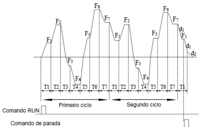
Fig.6-42 CLP em modo contínuo
