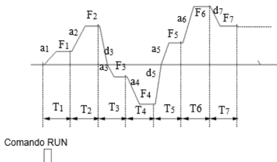
Fig.6-41 CLP operando na frequência final
