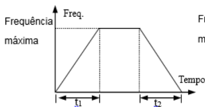
Fig.6-4 Acel./Desacel. linear
