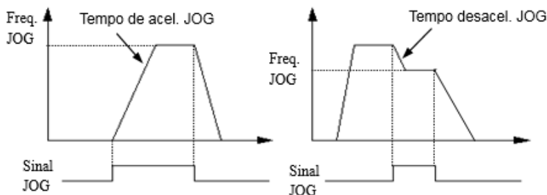
Fig.6-14 Função JOG
