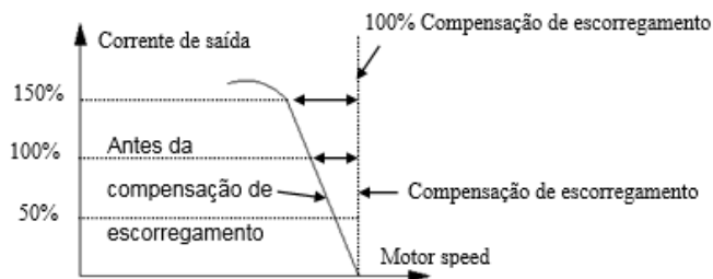
Fig.6-13 Compensação da freq. de escorregamento
