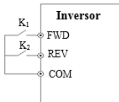
Fig.6-21 Comando 2 fios modo 1
