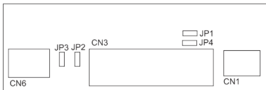
Fig. 3-7 Posição dos conectores e jumpers (Inversores acima de 7,5kW)
