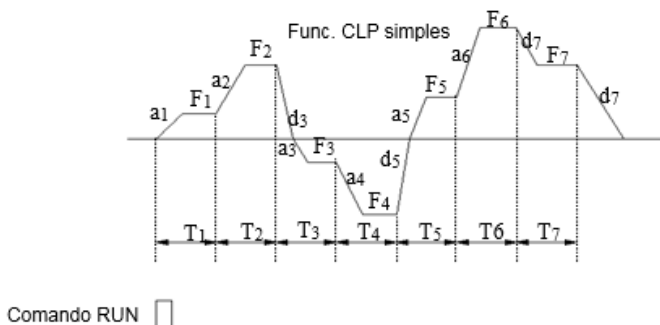
Fig.6-40 O CLP para após um ciclo simples
