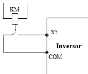
Fig. 6-20 Falha externa normalmente aberto
