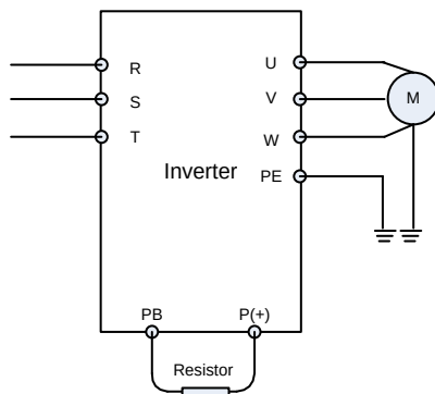
Fig.2-2 Conexão do resistor de frenagem
