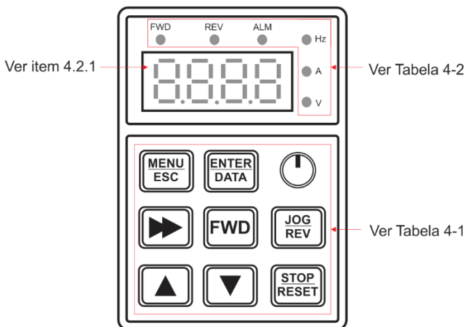
Fig. 4-1 Painel de controle (IHM até 1,5kW 220V)
