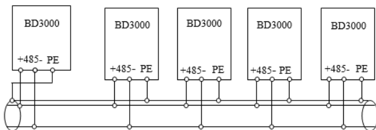
Fig. 3-12 Comunicação mestre-escravo multi inversores.
