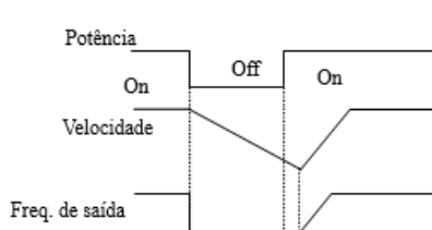
Fig.6-9 Detecção de velocidade
