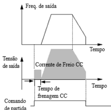
Fig.6-11 Modo de partida 1
