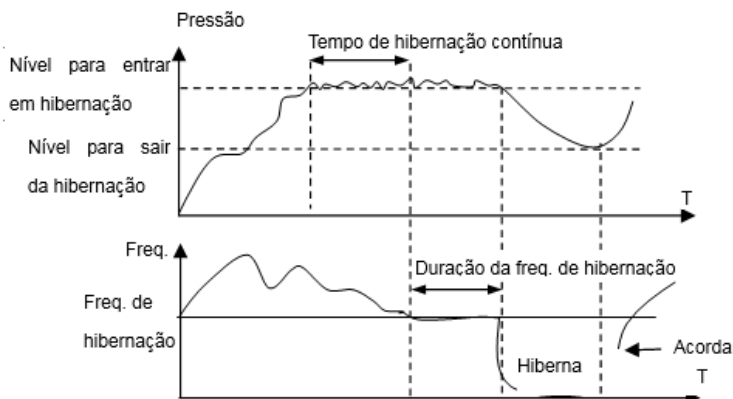
Fig.6-34 Entrada e saída do modo de hibernação
