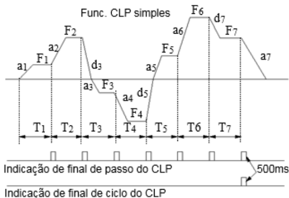
Fig.6-39 Modo CLP simples
