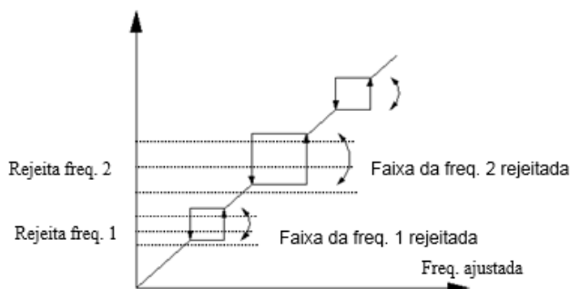
Fig.6-15 Freq. e Faixa de frequência rejeitada
