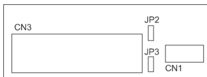
Fig. 3-5 Posição dos conectores e jumpers (Inversores até 1,5kW 220V)
