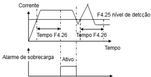
Fig. 6-29 Alarme de sobrecarga
