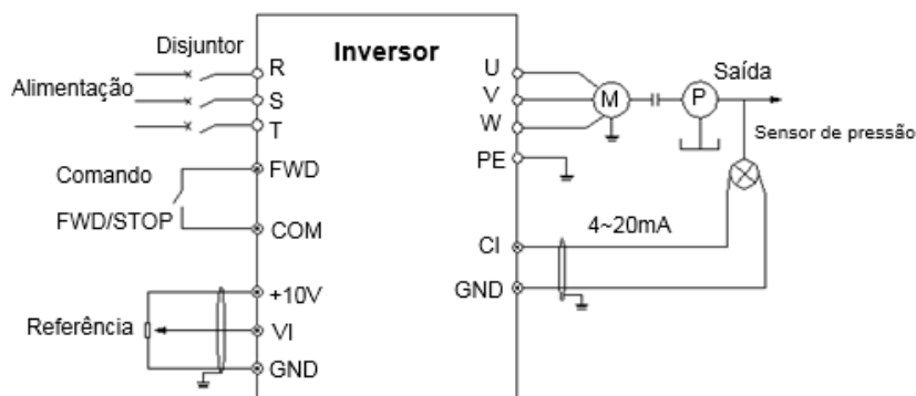
Fig. 6-32 Controlador PI com realimentação analógica
