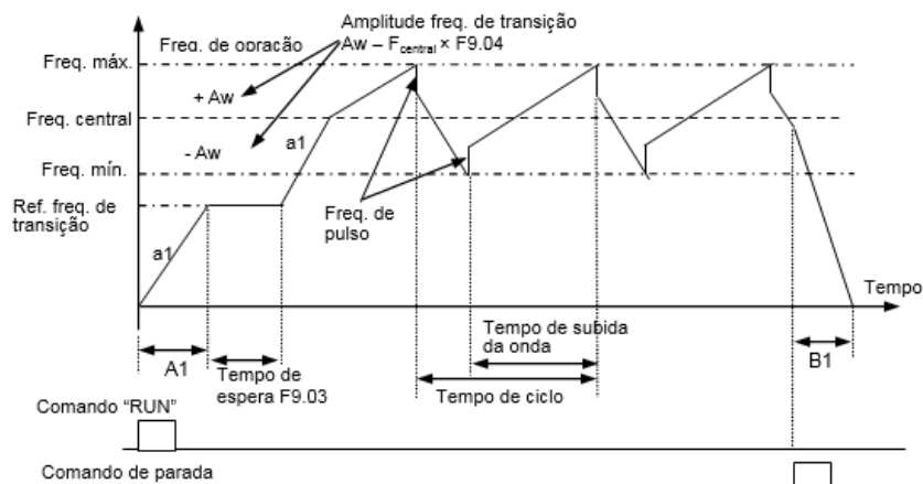
Fig.6-44 Função de transição
